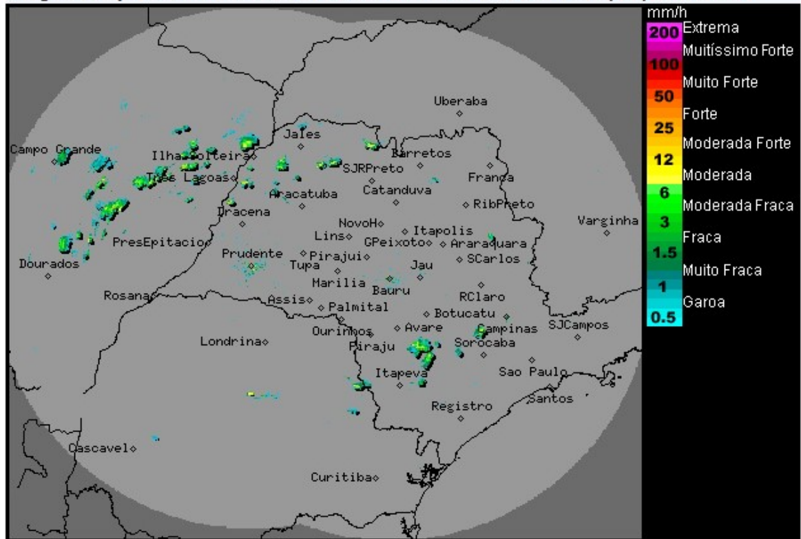
Imagem Composta dos Radares de Bauru e de Presidente Prudente - 25/03/2017 16:45
