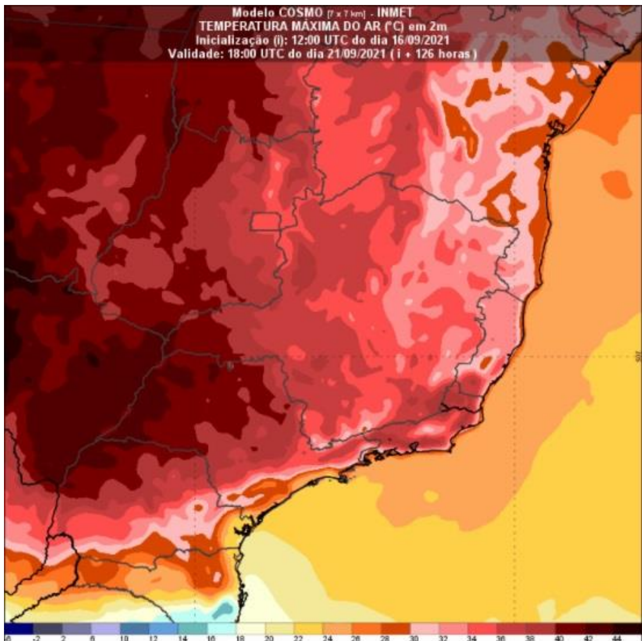
Figura 1 – Simulação do modelo COSMO/INMET com a temperatura máxima.
